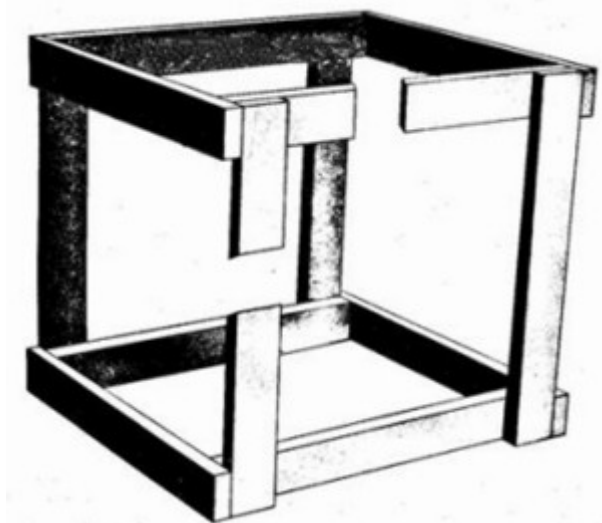
FIGURA 3. Un posible modelo de una canasta imposible
